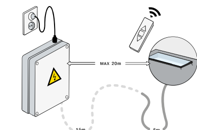
7. Schließen Sie die beiden Kabel im Inneren gemäß beiliegendem Plan an. Platzieren Sie das Schaltbrett an einem gut zugänglichen Ort (z. B. Zählerschrank).
