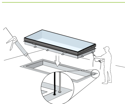
4. Tragen Sie Dichtungsmasse auf und führen Sie beim Absenken beide Stromkabel durch die vorbereiteten Löcher.
