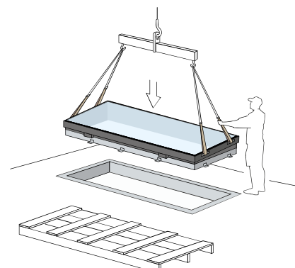
3. Auf dem Dach von der Palette los-schrauben und über die Aussparung heben
