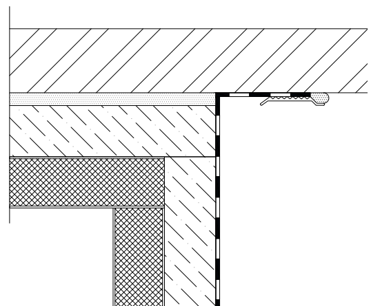
Draufsicht: Anschluss Dachabdeckung
